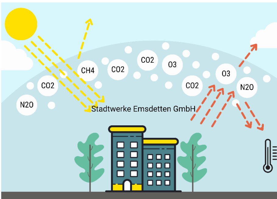
Abbildung 1 - Der Treibhauseffekt
